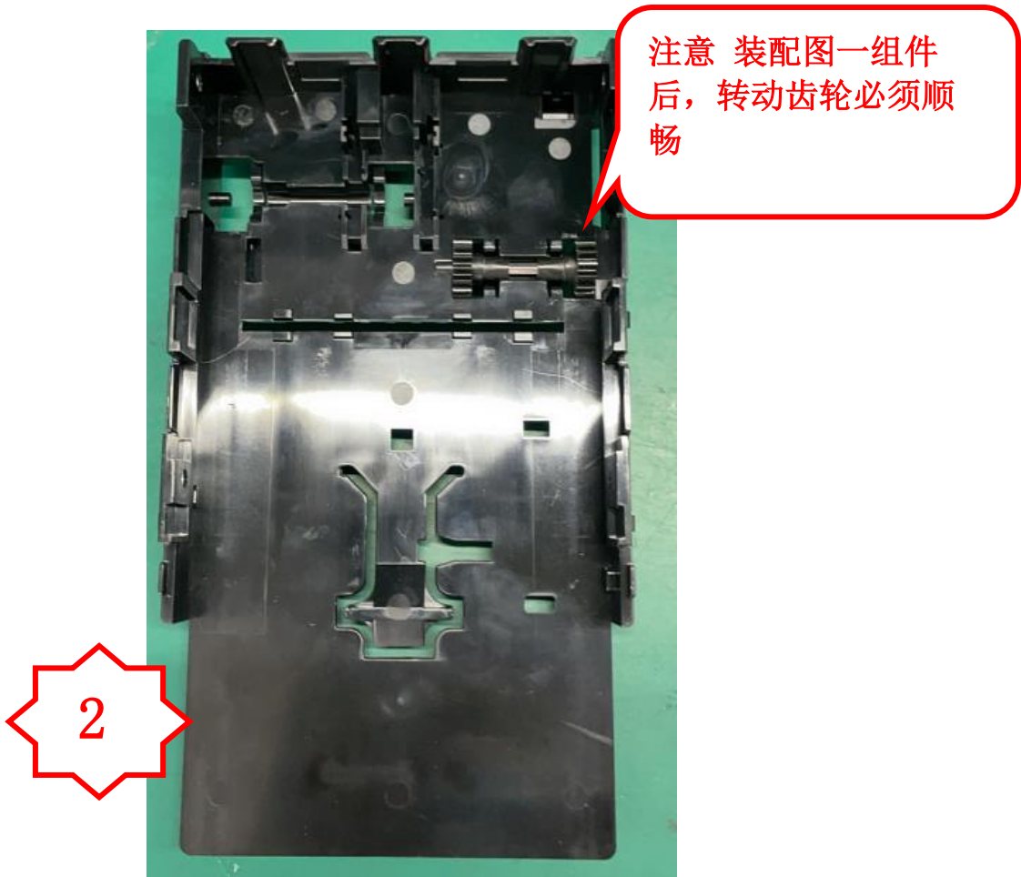
图二，将图一组件如图卡在 PM2626 上
