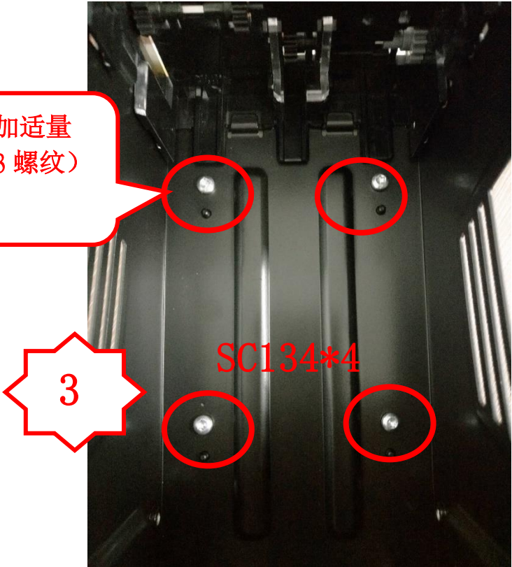
图三, 将 PA2740-7 放入治具中, 将四颗 SC134 加螺纹胶打在正确的位置
