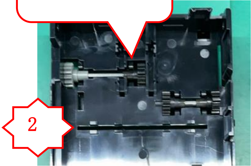
图二，将图一组件如图卡在 PM2626 上，注意方向
